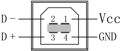
图 5-3 USB 串口
