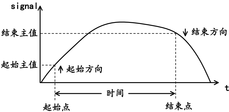
图 3-39 时间测量功能
