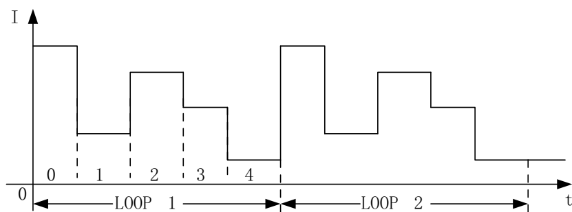
图 3-19 序列波形
