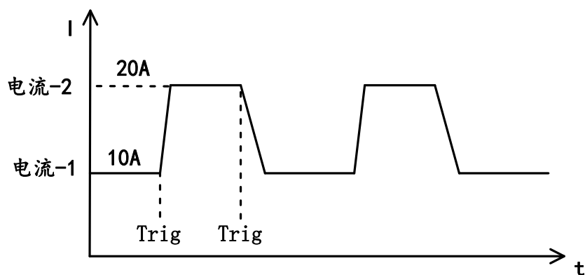
图 3-12 翻转模式
