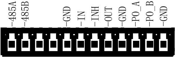
图 5-2 RS485 串口
