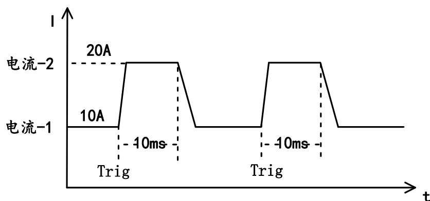
图 3-11 脉冲模式
