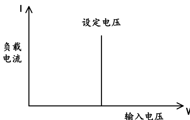
图 3-4 定电压模式
