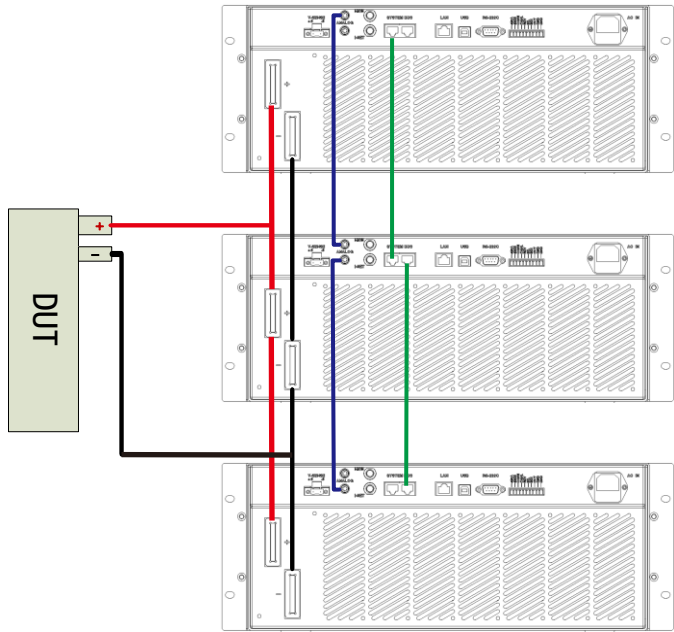
图 3-35 并机接线
